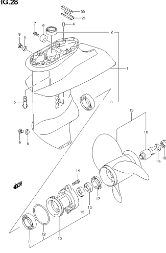
DF15A 20A P01 013_G68 GEAR CASE
