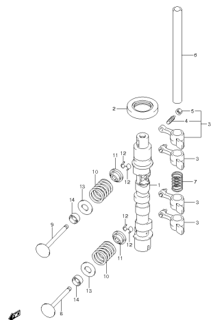
DF15A 20A P01 013_005 CAMSHAFT
