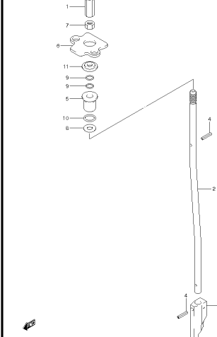
DF15A20A P01 013_016 SHIFT ROD
