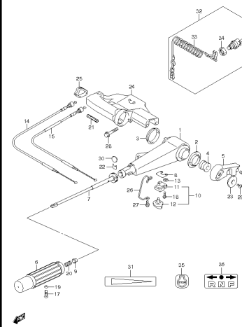
DF15A 20A P01 013_G82 TILLER HANDLE
