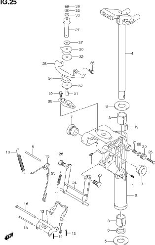
DF15A 20A P01 013_G65 SWIVEL BRACKET
